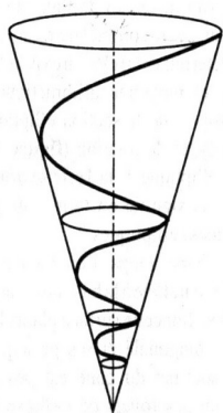
Figure 2. Une spirale logarithmique sur un cône.
